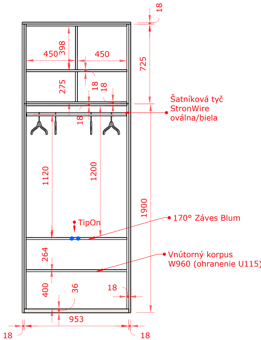
Pohl'ad spredu
