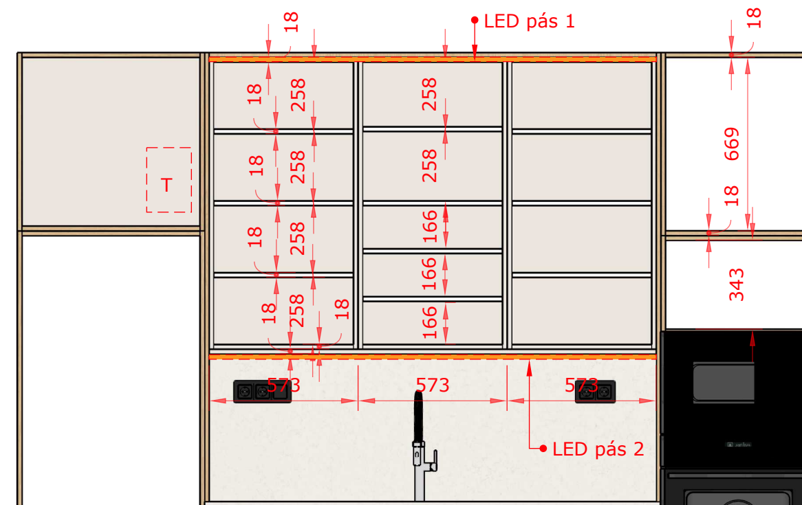
Pohl'ad spredu
